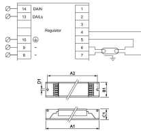
Technische Daten Philips HF-Ri TD 1 28/35/49/54 TL5 E+ 195-240V
